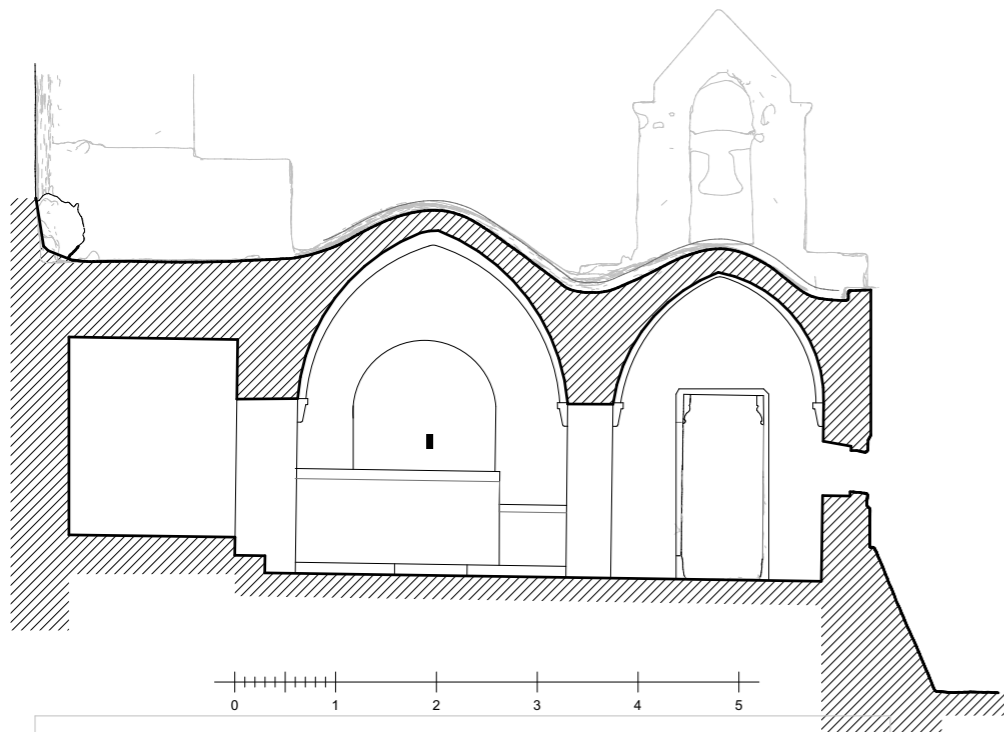
ΤΟΜΗ Τ2-2'
